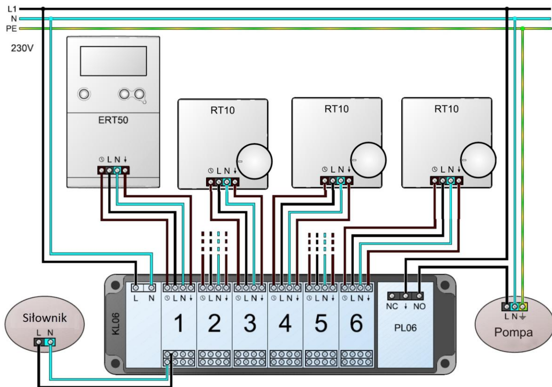
Schemat podłączenia – 3 żyłowy przewód bez funkcji NSB
